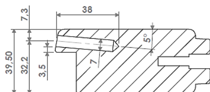
COUPE B-B ECHELLE 1 : 2
