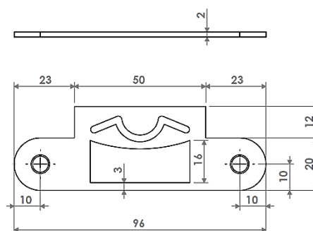
Gâche haut/bas ROZ 3 pts
