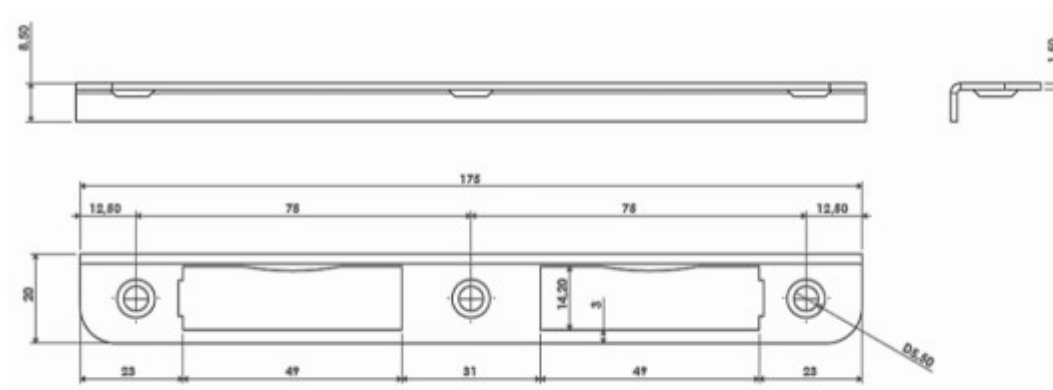
Gâche serrure standard ROZ
