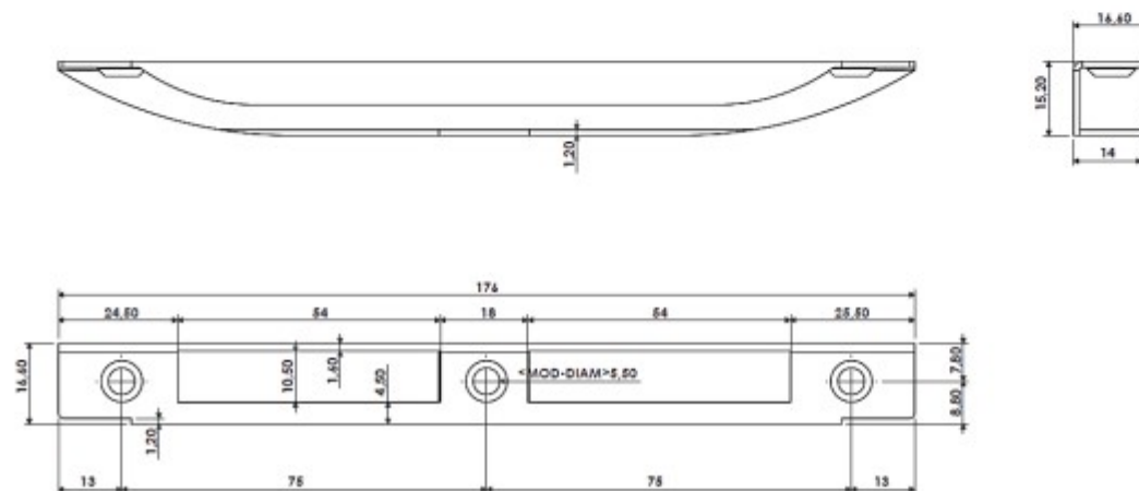
Gâche serrure standard OLT
